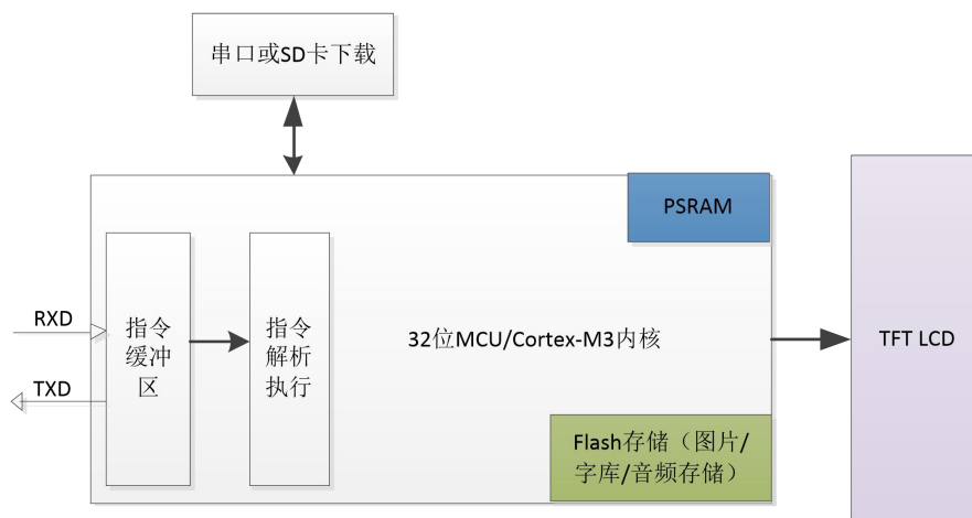
图 2-1 S 系列串口屏内部结构图
