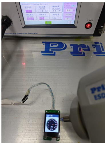
图 5-2 ESD 测试图
