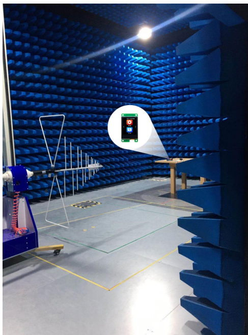
图 5-5 辐射测试图
