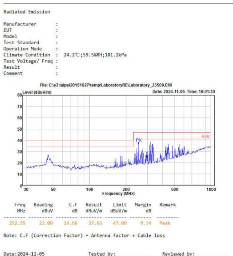
图 5-7 辐射测试垂直方向
