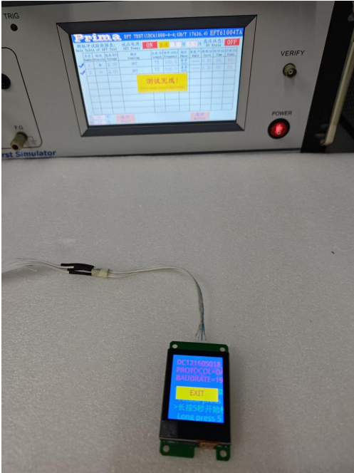
图 5-4 群脉冲测试图
