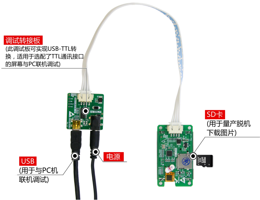
图 1-3 调试工具图
