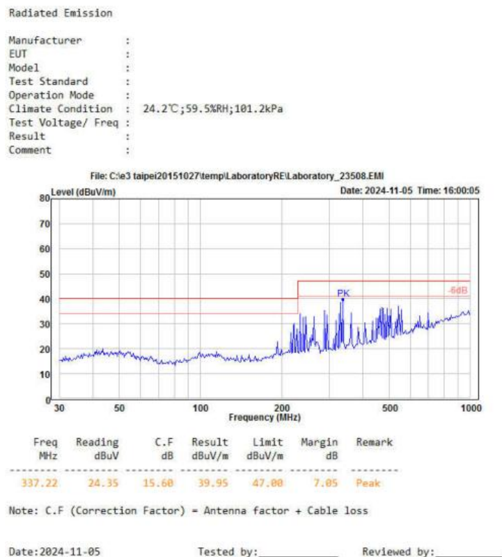
图 5-6 辐射测试水平方向
